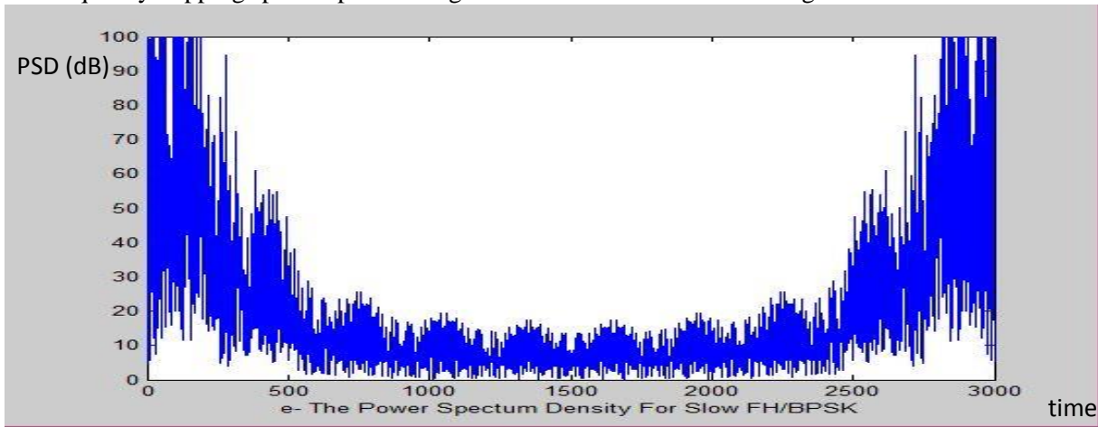
Figure.7 The Slow FH/BPSK result plots
